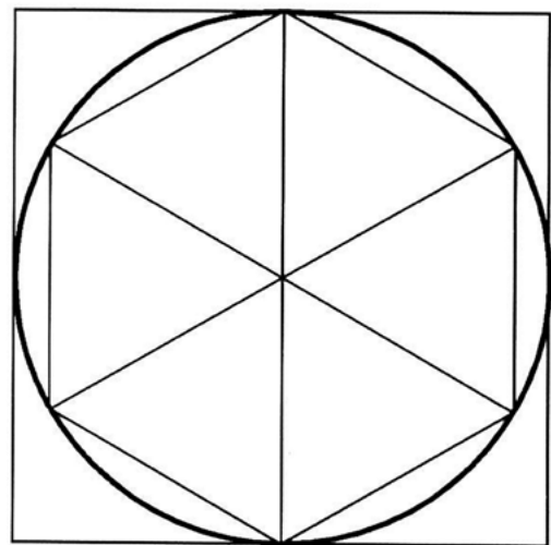
Abb. 6. Kreisumfang-Näherung (HOLE, 1998, 72)
